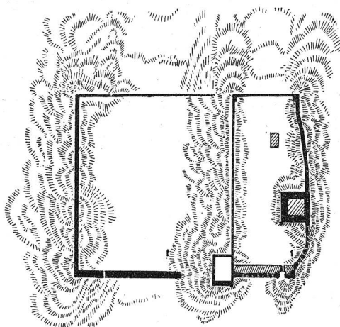
Slika 3. Tlocrt Ključa (Stevan R. Delić, Dva stara natpisa iz Hercegovine, Glasnik Zemaljskog muzeja u Bosni i Hercegovini , 23/1911, str. 492) / Figure 3. Ground plan of Ključ
